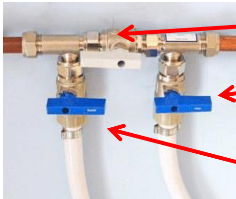
Voorbeeld externe bypass
